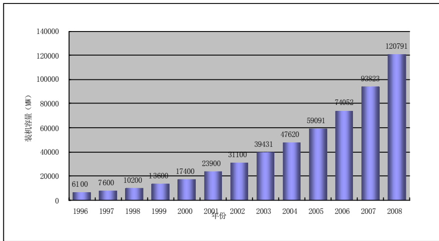
1996—2008 年全球总装机容量
