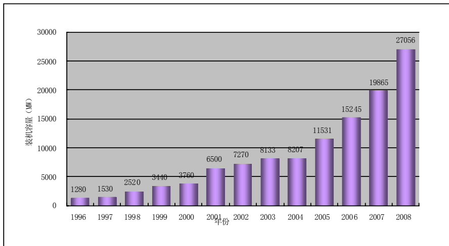
1996—2008 年全球每年新增装机容量
