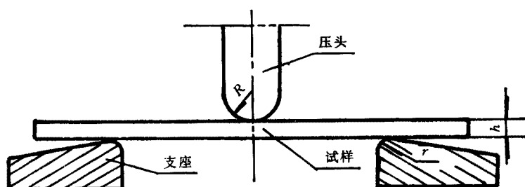
图 1 试样、加载压头和支座示意图
