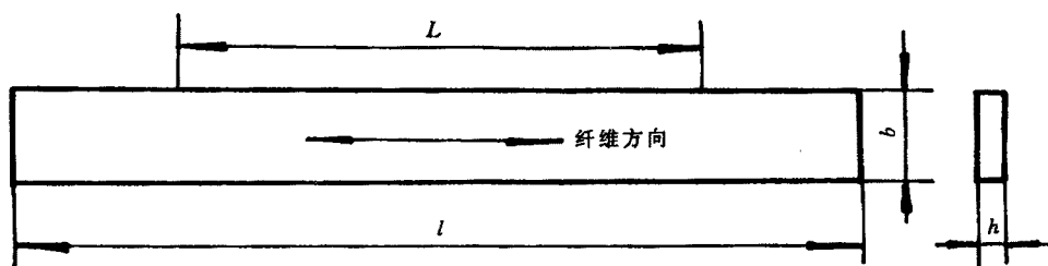
l —试样长度; L —跨距; b —试样宽度; h —试样厚度
