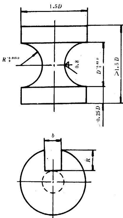
图 1 支承点尺寸
