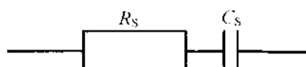
串联等值电路
